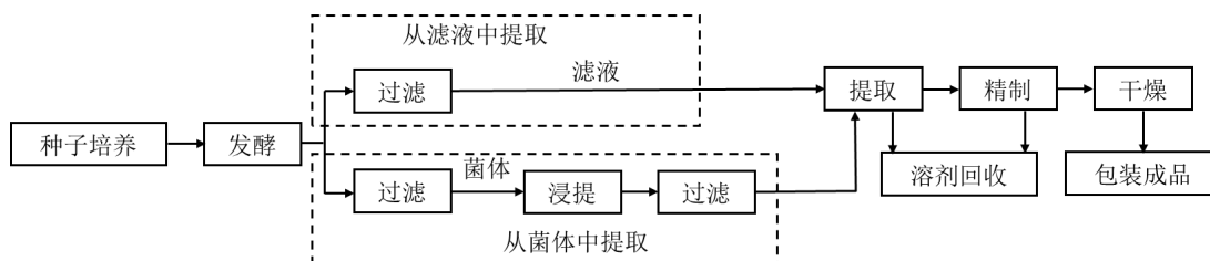
图 26-1 发酵制药生产工艺流程图
