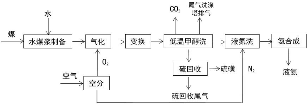
图 25-1 水煤浆气流床气化工序合成氨生产工艺流程图
