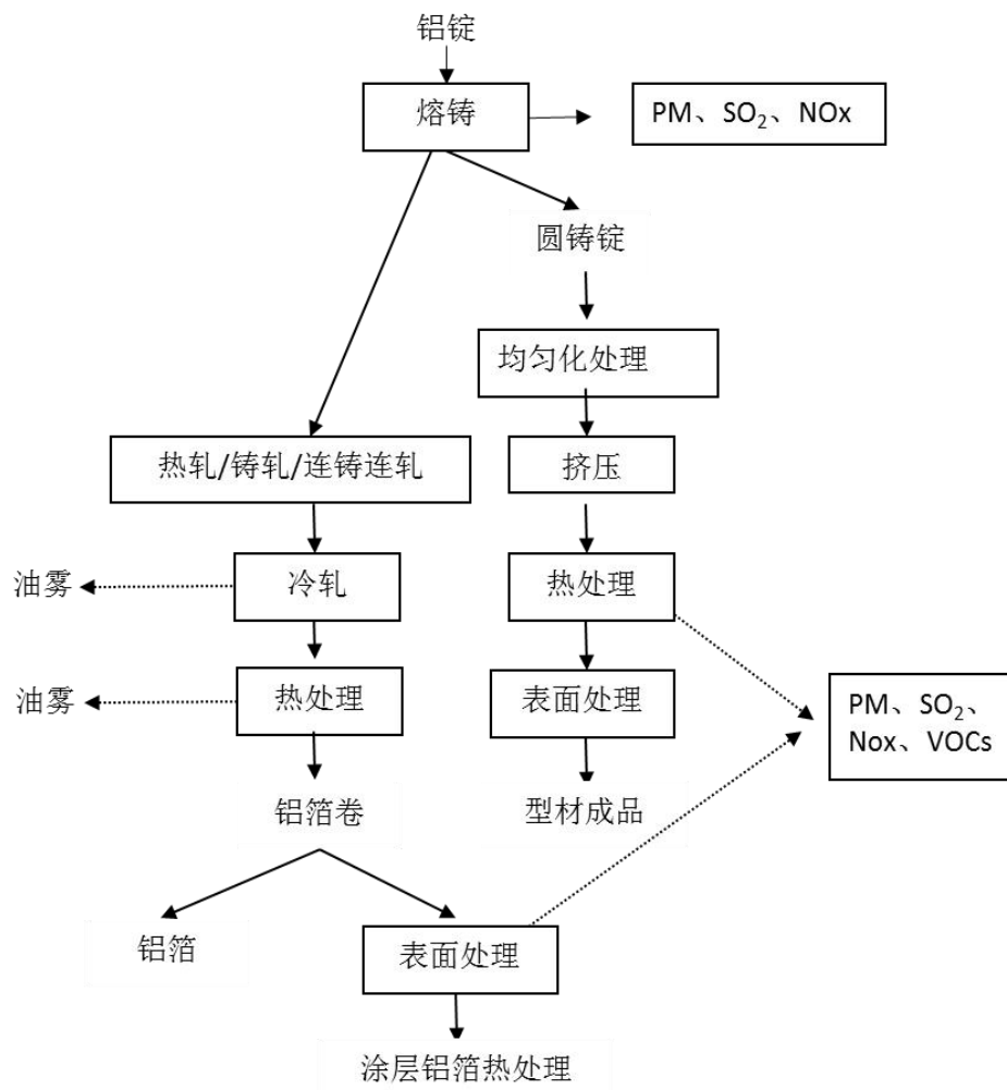
图 14-2 铝板带箔及型材典型生产工艺流程图
