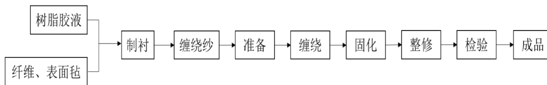
图 21-1 缠绕生产工艺流程图
