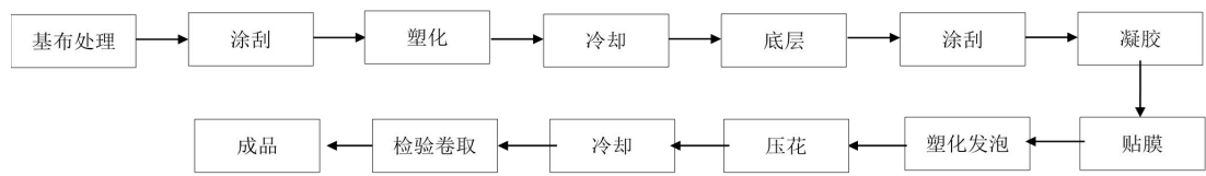
图 33-1 聚氯乙烯直接涂刮法生产工艺流程图
