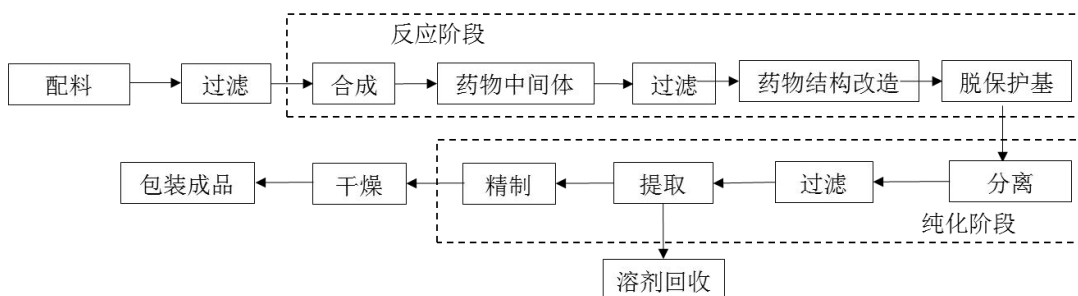
图 26-2 化学合成制药生产工艺流程图
