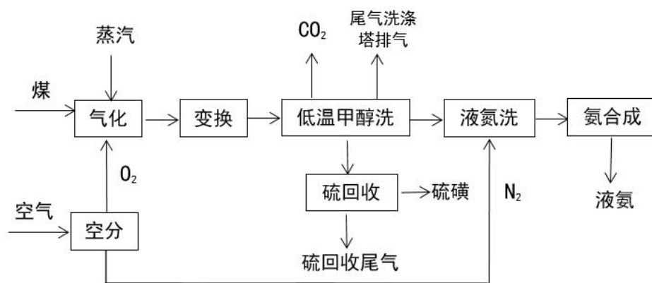
图 25-3 碎煤固定床加压气化工工艺合成氨生产工艺流程图
