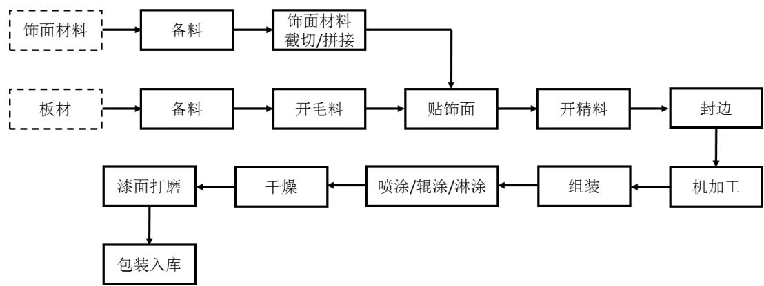
图 36-2 典型板式家具制造生产工艺流程图
