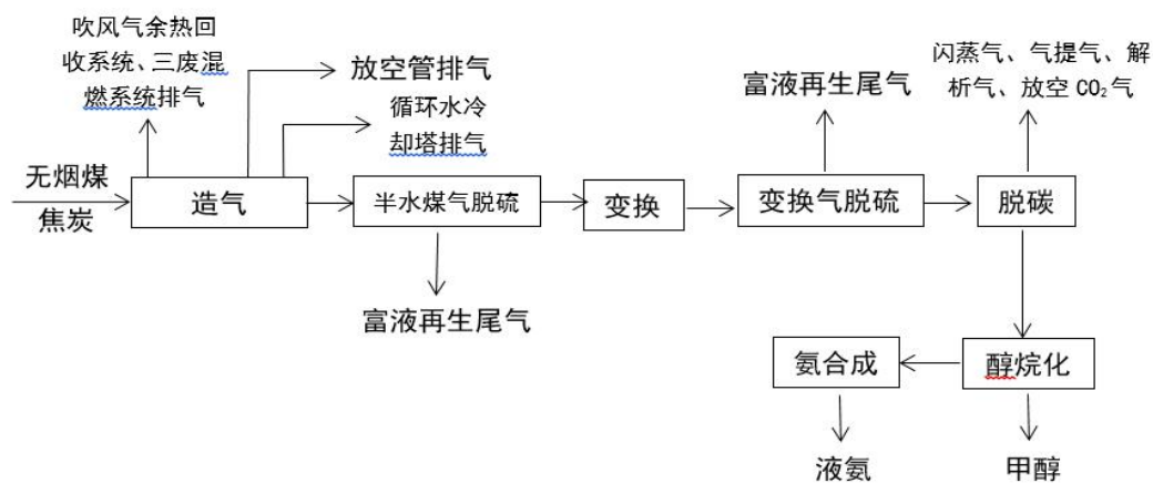
图 25-4 固定床常压间歇煤气化工工艺合成氨生产工艺流程图
