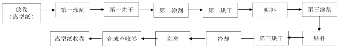
图 33-4 聚氨酯干法工艺生产工艺流程图
