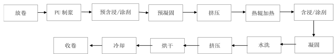
图 33-5 聚氨酯湿法工艺生产工艺流程图
