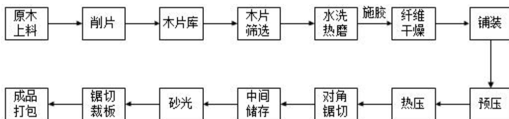
图 32-3 纤维板制造生产工艺流程图
