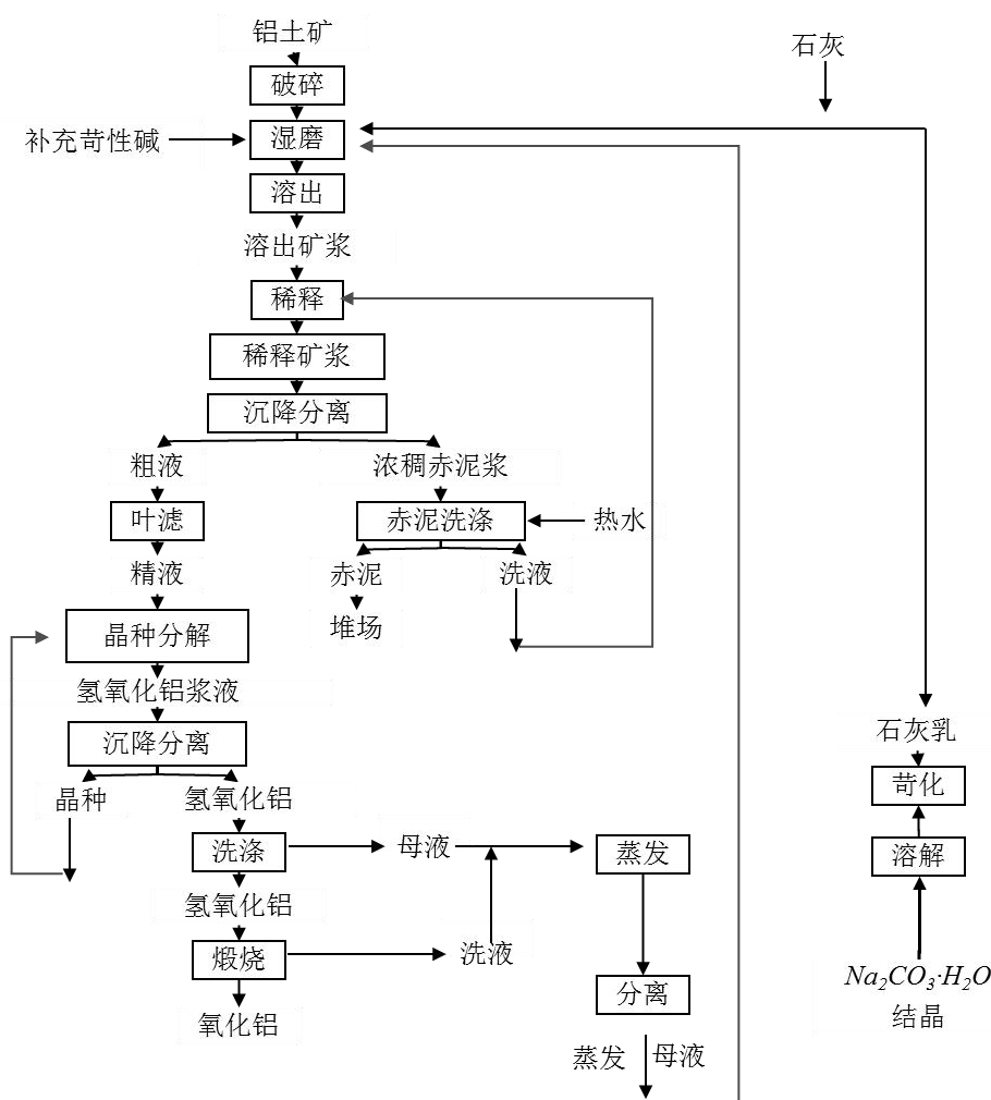
图 7-1 典型拜耳法氧化铝生产工艺流程图
