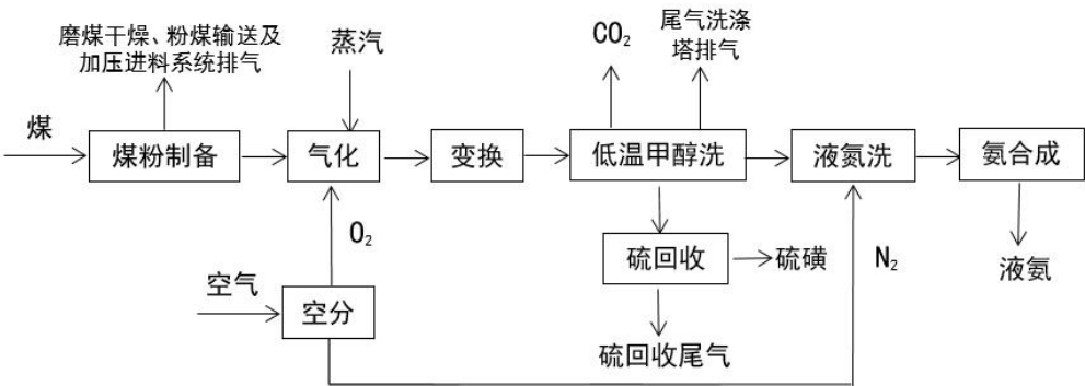
图 25-2 干粉气流床气化工序合成氨生产工艺流程图
