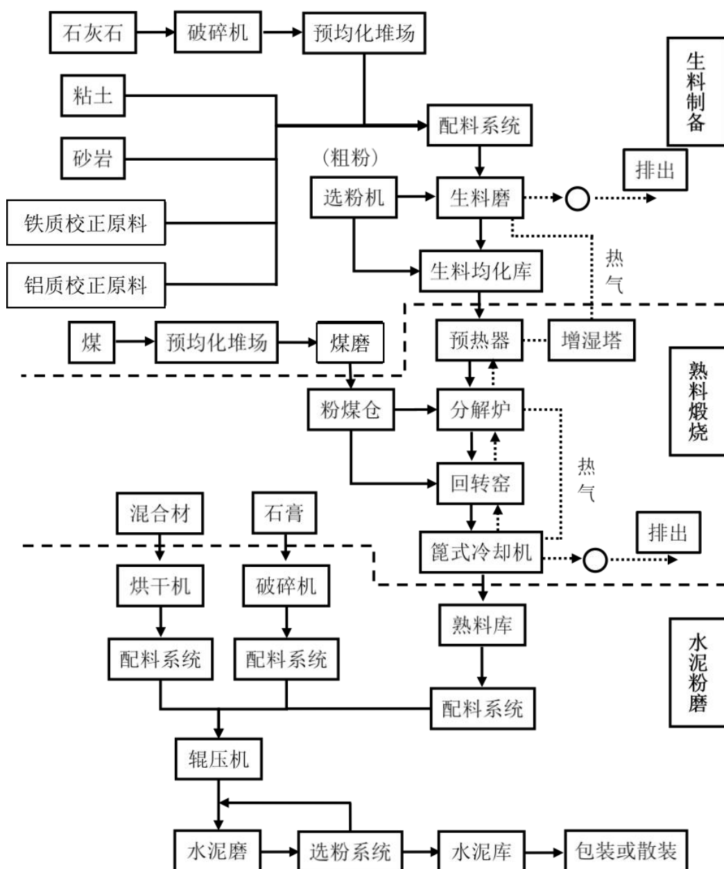
图 15-1 典型水泥制造生产流程图
