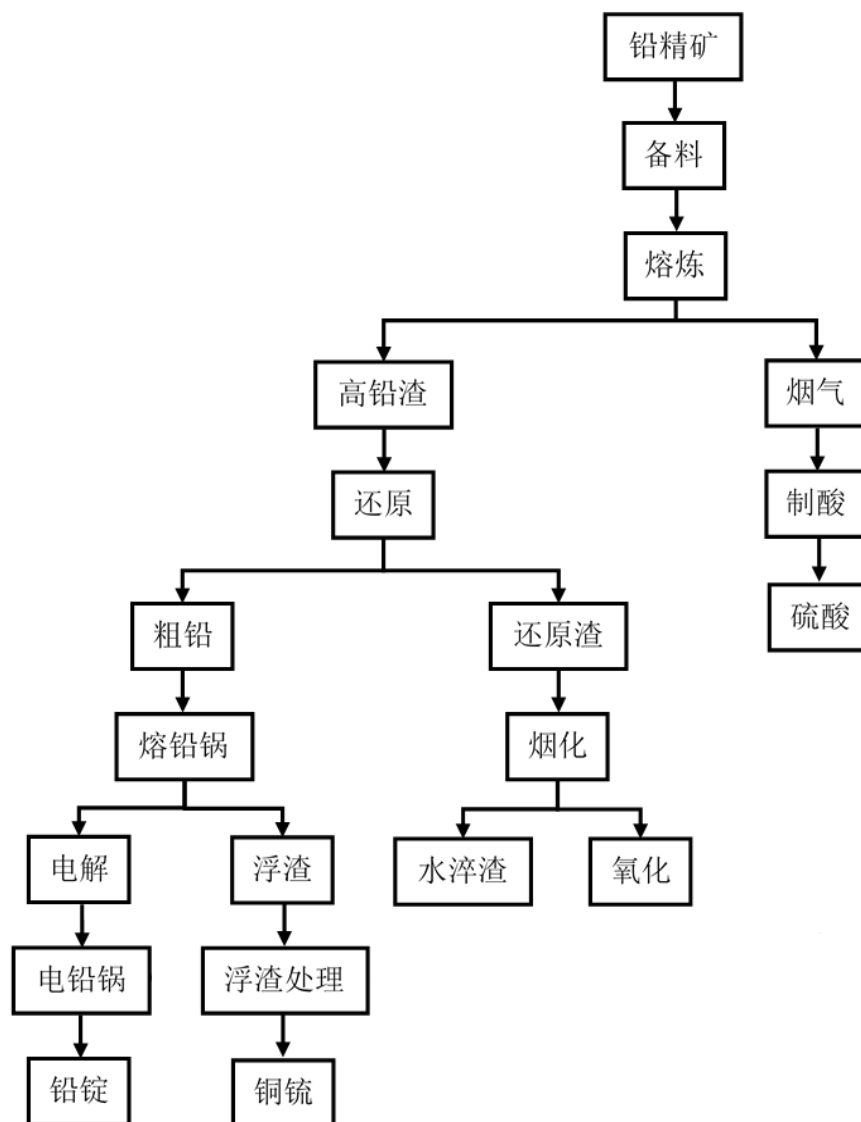
图 11-1 铅冶炼典型生产工艺流程图
